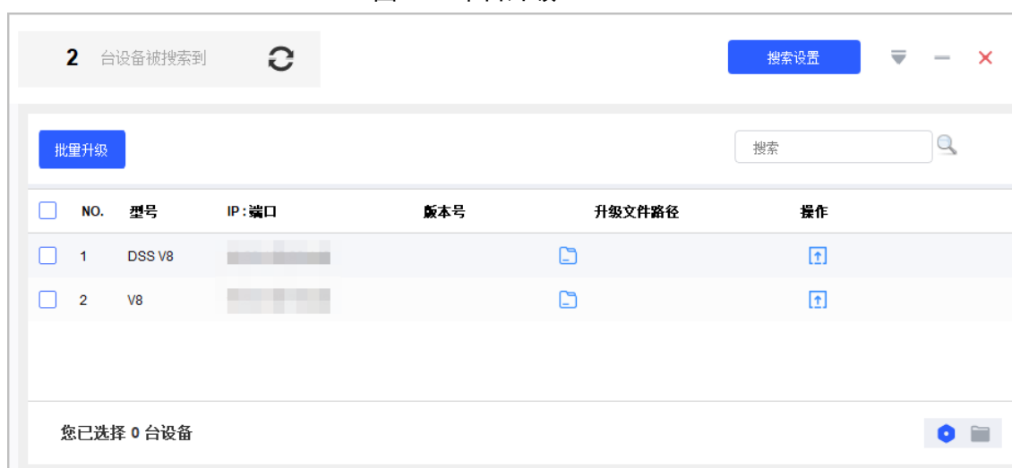
图4-11 单台升级
