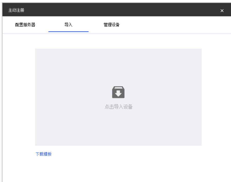
图4-3 下载模板
