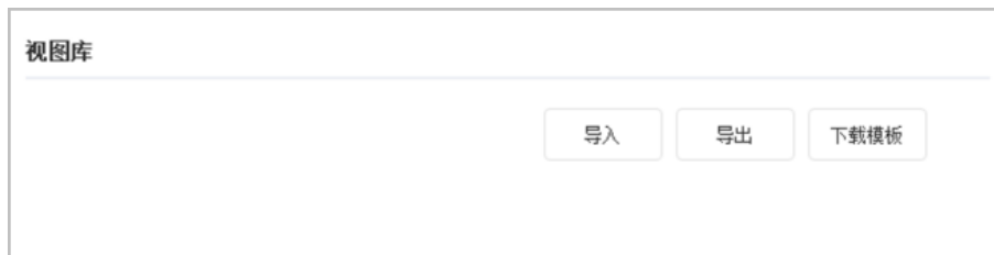
图4-73 视图库配置
