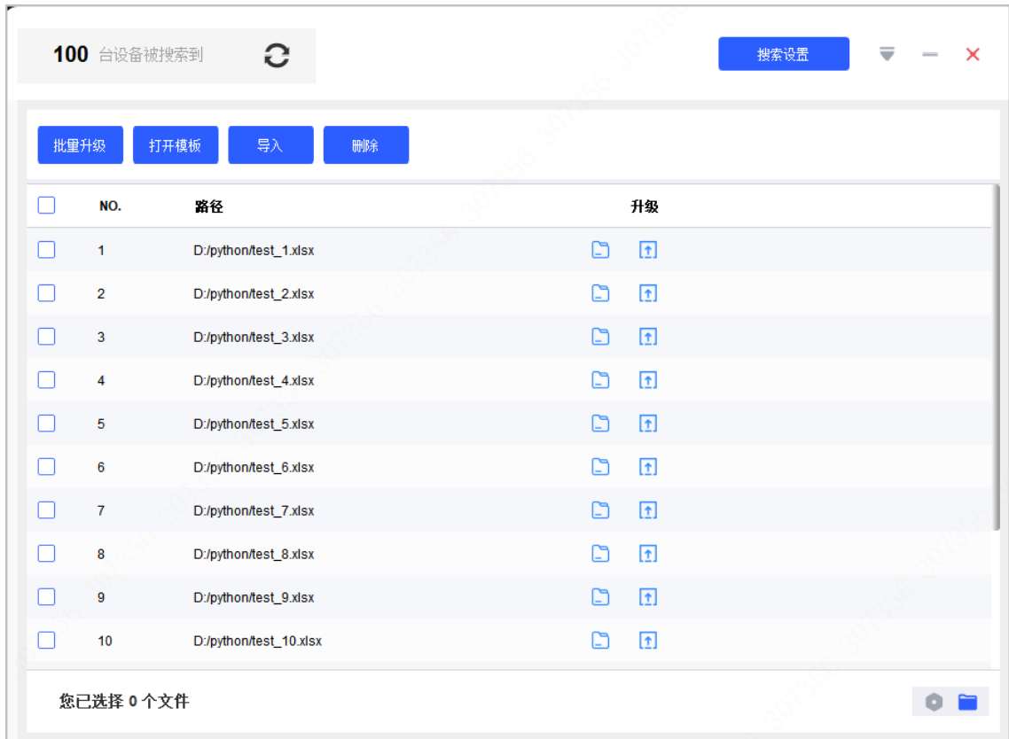
图4-13 文件升级
