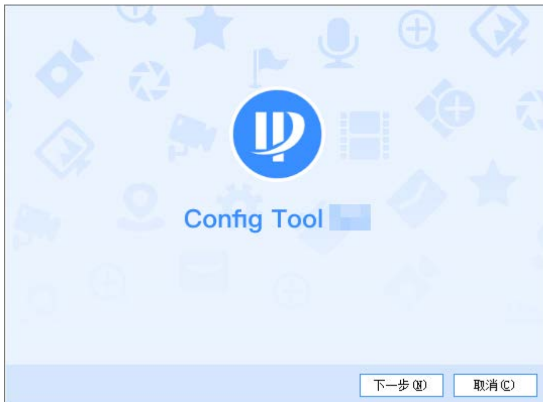
图2-2 安装工具
