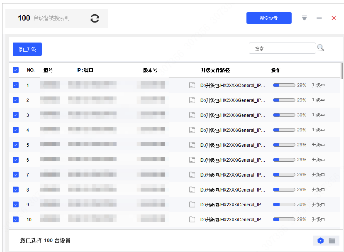
图4-12 批量升级
