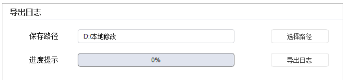
图4-50 导出日志
