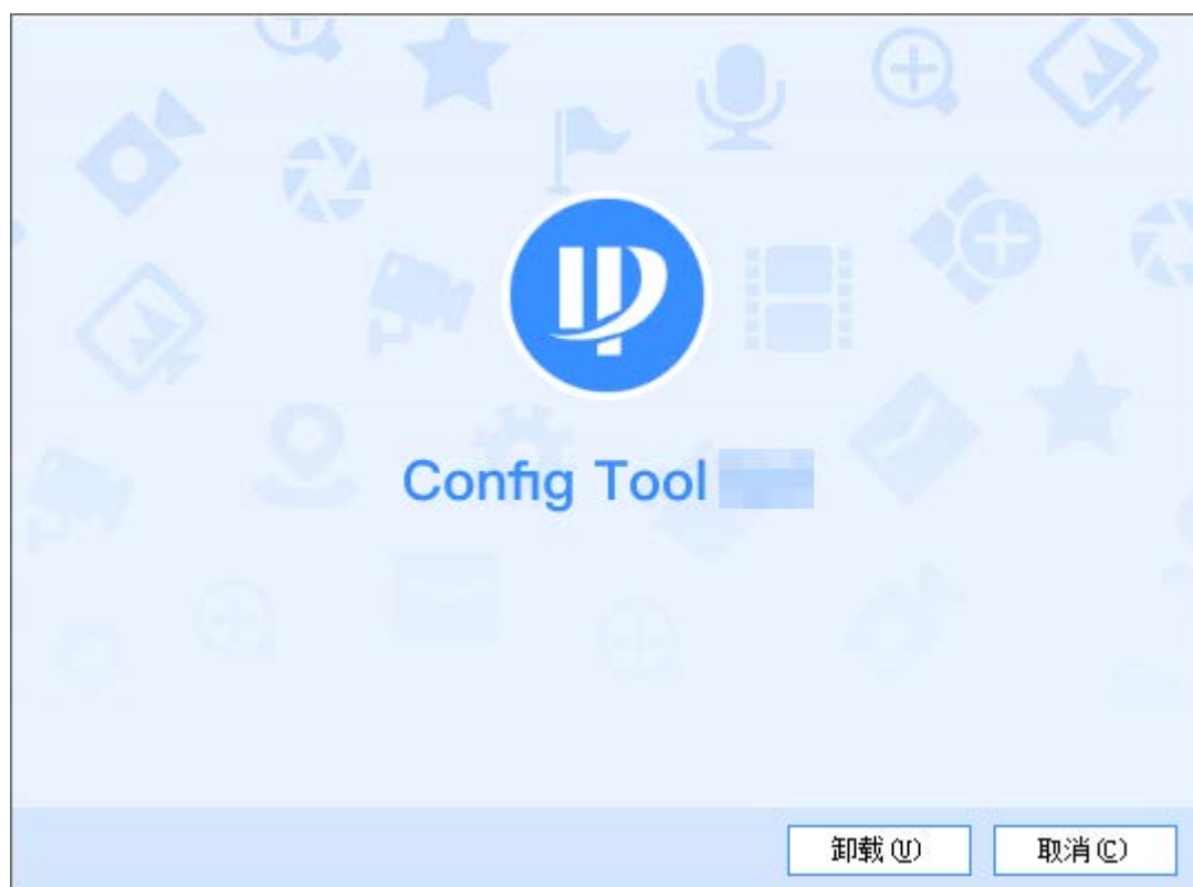
图2-8 卸载工具
