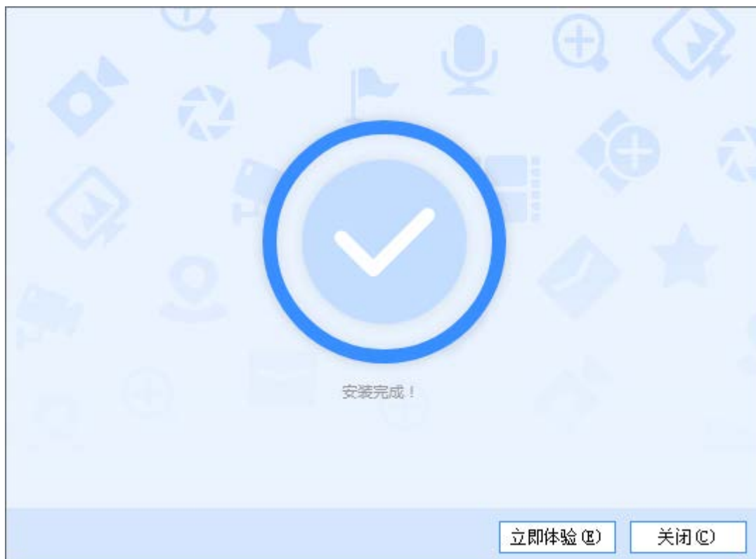
图2-3 安装完成
