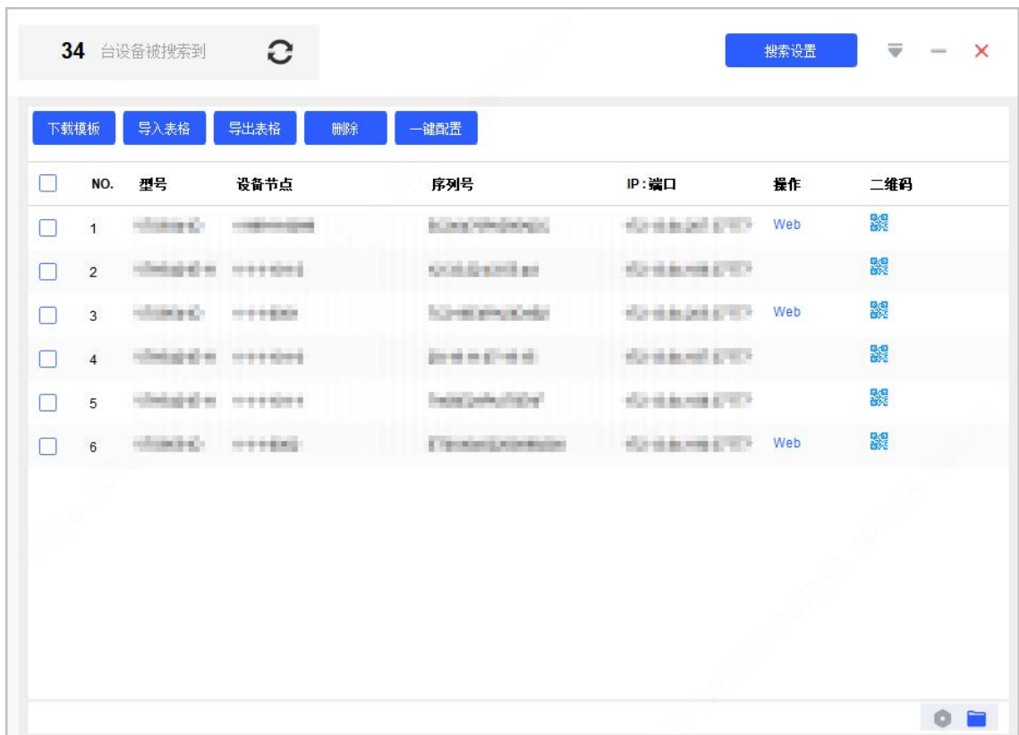
图4-84 导入配置
