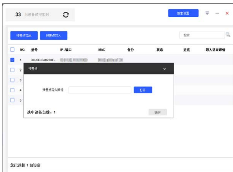
图4-91 导入预置点
